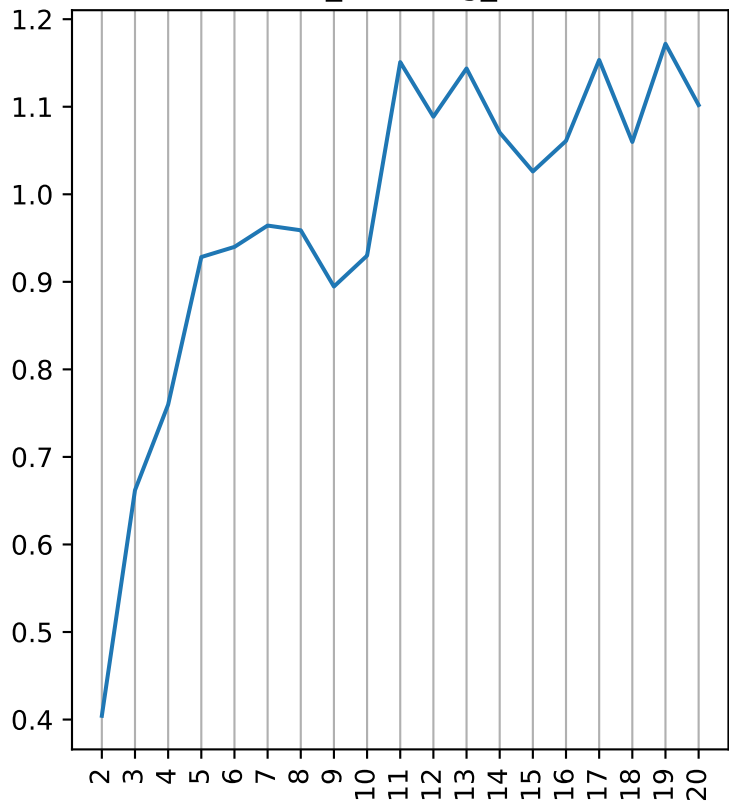
Davies_boulding_score
